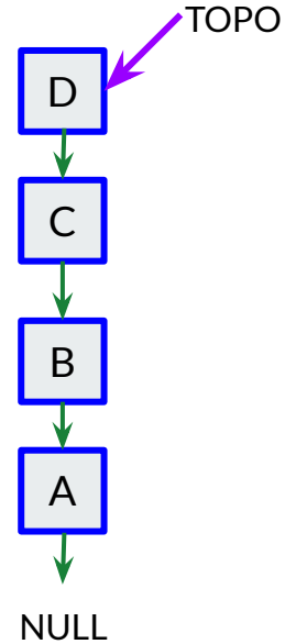
Pilha Dinâmica (Lista Ligada)
